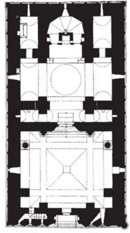
Աղբակի Ս. Բարդուղիմեոս վանքի հատակագիծը
