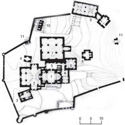
Հաղպատի վանքի հատակագիծը. 1. Ս. Նշան եկեղեցին, 2. գավիթը, 3. Ս. Գրիգոր եկեղեցին, 4. Ս. Աստվածածին մատուռը, 5. տապանատուն, 6. գրատուն, 7. «Համագասպի ժամատունը», 8. զանգակատուն, 9. սեղանատուն, 10. Ուքանանց տոհմի դամբարանները, 11. մուտքեր
