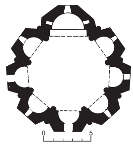
Եղվարդի Ս. Թեոդորոս վանքի եկեղեցու հատակագիծը
