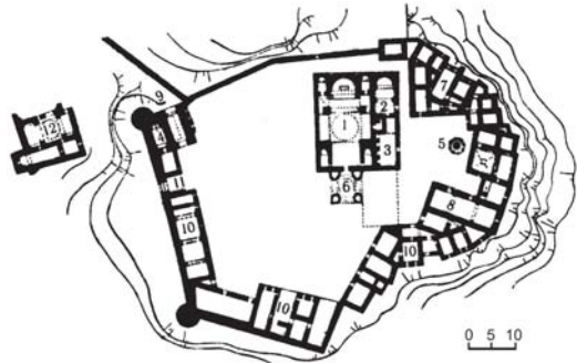
Տաթևի վանքի հատակագիծը. 1. Ս. Պողոս-Պետրոս տաճարը, 2. Ս. Գրիգոր Լուսավորիչ եկեղեցին, 3. սրահը, 4. Ս. Աստվածածին եկեղեցին, 5. «Գաղազան» հուշատունը, 6. դանգակատունը, 7. առաջնորդարանը, 8. սեղանատունը, 9. դարպասը, 10. բնակելի և տնտեսական շինությունները, 11. աղբյուրը, 12. ձիթհանը
