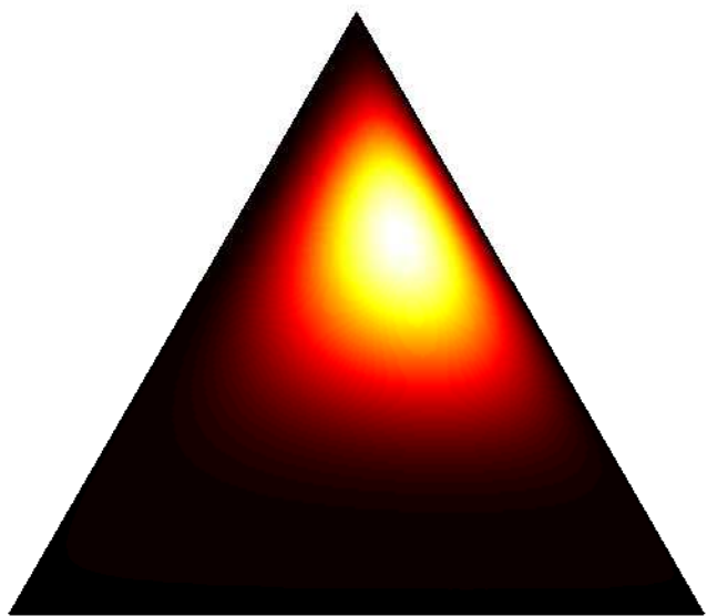
Dirichlet
