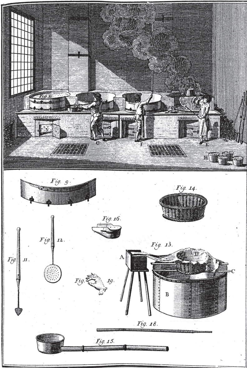
Afbeelding van eenige voornaame verrichtingen en gereedschappen in de Raffinaderij. (uit: Reisig, De suikerraffinadeur) Fig. 9 Een groot Voorzetsel. Fig. 10 Een klein Voorzetsel op het groote voor de pan geplaatst. Fig. 11 Een spitskrabber. Fig. 12 Een Schuimspeen. Fig. 13 Een Stremijnlaken. A is de Bak of Stoel van het Laken. B De Klaarselketel. C De ijzeren Burrie. D De Klaarselmand met het Laken bekleed. Fig. 14 De Klaarselmand. Fig. 15 Een koperen Buis, door welke men het klaarsel uit den ketel in den mand laat lopen. Fig. 16 Een Afdraagbekken. Fig. 17 Een Candybekken met water op den Furnuis der pannen. E De Meester die bezig is de Zeede aanteproeven. F Een Werkman, die met een roerhout in de pan roert. G Een ander, die schuimt. Fig. 18 Een proefstok. Fig. 19 Eene hand, welke de proef neemt. Fig. 22 Een omgekeerde Candijpot op de pannen. H Eenige afgedompte Candijpotten.
