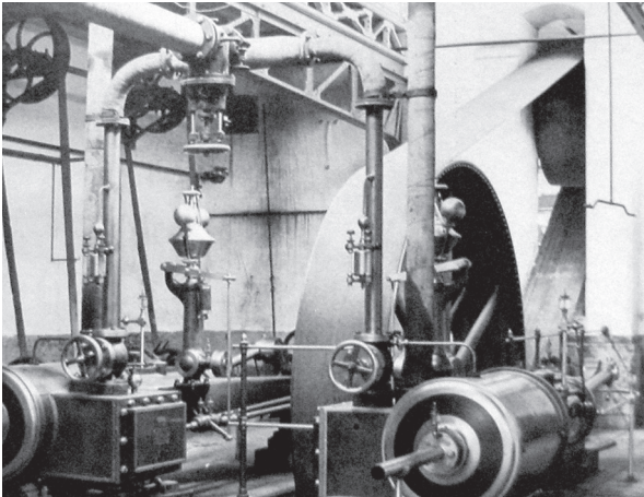
Stoomaangedreven drijfmachine die wel een tiental suikercentrifuges kon aandrijven (afb.: archief Suiker Unie).
