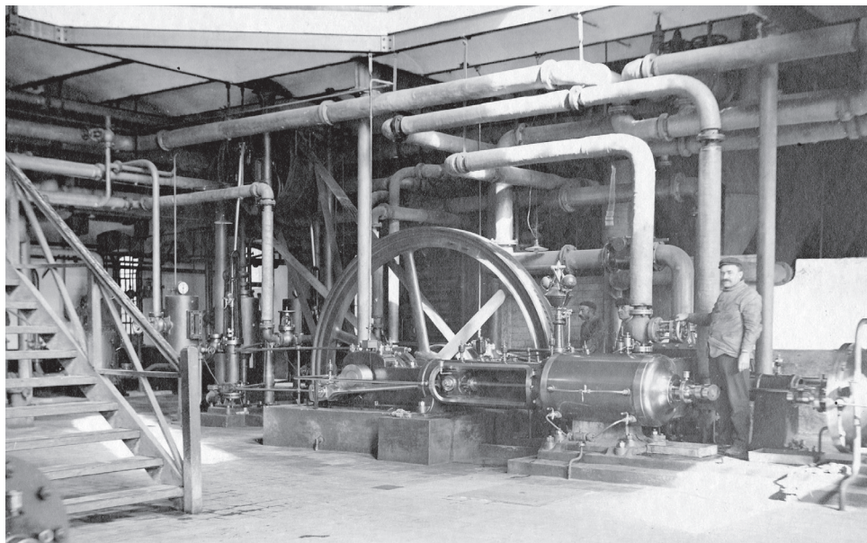
Door stoom aangedreven koolzuurgaspomp ENCB 1910 (afb.: archief Suiker Unie).
