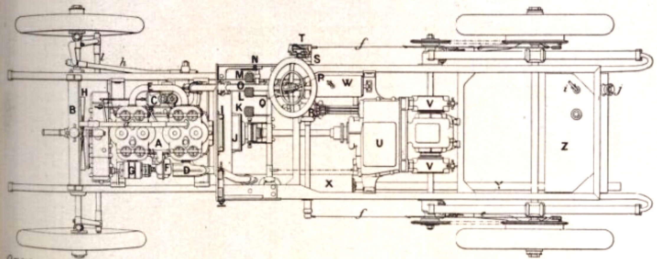
Fig. 8. — CHASSIS WESTINGHOUSE 1907, DE 35-40 CHEVAUX. — A, moteur. — a, tuyauterie de retour d'eau — B, radiateur. — C, carburateur. — D, pompe à eau. — E, soupapes. — F, pistons. — G, bielles. — H, volant. — I, manivelle. — J, embrayage. — K, boîte de vitesses. — L, arbre. — M, frein. — N, tambour. — O, levier de frein. — P, pédale de frein. — Q, câble de frein. — R, tambour. — S, tambour. — T, tambour. — U, transmission. — V, axe. — W, axe. — X, châssis. — Y, châssis. — Z, axe arrière.
