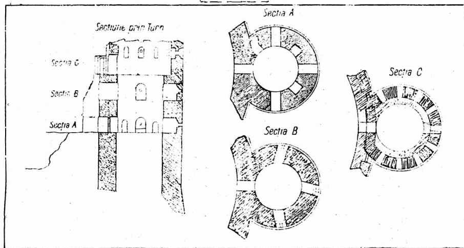
Detalii SCARA 1/50
